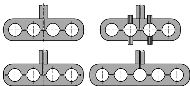
Рис. 1. Схемы многопозиционных индукторов
