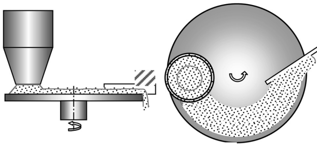
Рис. 3. Тарельчатый дозатор
