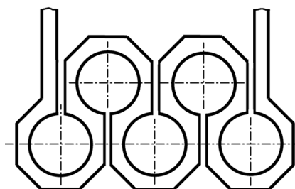
Рис. 2. Схема многогнездного индуктора по А.с. СССР 909852
