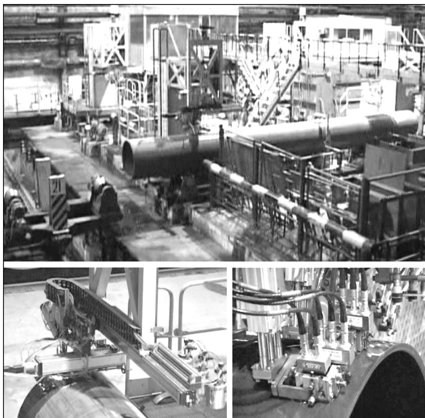
Рис. 1. Установка НК 362М в ТЭСЦ-4 ОАО «Выксунский металлургический завод»
