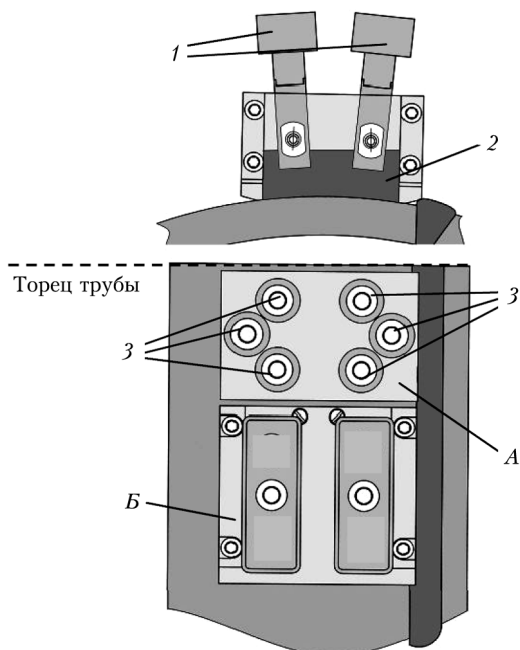
Рис. 2. Схема контроля и пространственное расположение ультразвуковых (УЗ) преобразователей: 1 — пленочные широкозахватные пьезоэлектронные преобразователи (ПЭП) фирмы «Krautkramer», зона контроля 60 мм; 2 — иммерсионная ванна; 3 — наклонные ПЭП с углом ввода 45°, зона контроля 30 мм; А, Б — акустические блоки для контроля наличия соответственно продольных дефектов и расслоений
